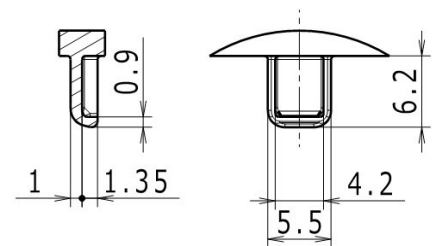
ストライカー形状 (参考)
