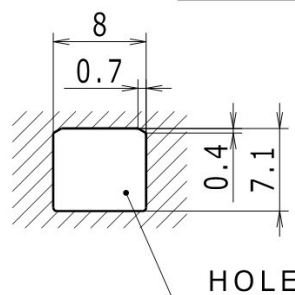
取付け穴形状 (参考)
